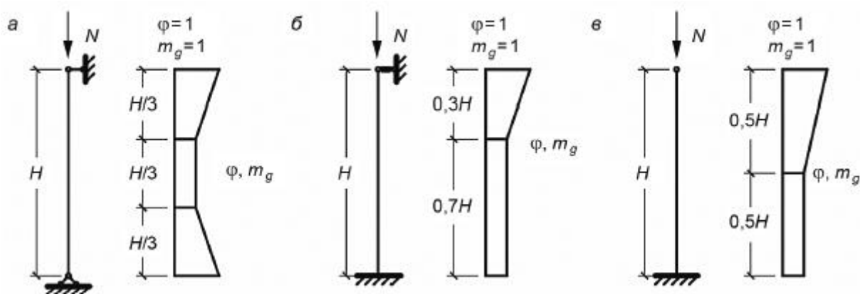
а - шарнирно опертых на неподвижные опоры; б - заземленных внизу и имеющих верхнюю упругую опору; в - свободно стоящих
