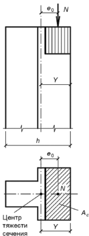
Рисунок 7.2 - Внецентренное сжатие
