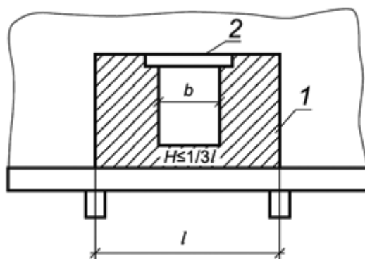
1 - нагрузка на рандбалку; 2 - железобетонная перемычка
