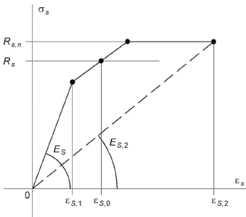
Рисунок Е.3 - Расчетная диаграмма деформирования стали
